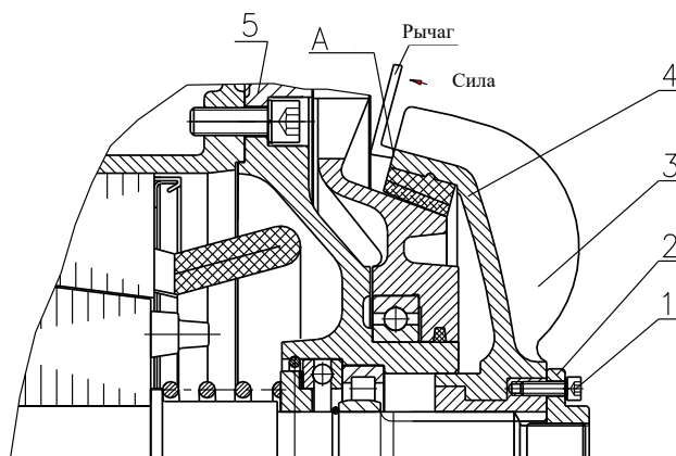
Тормозная система ТМ-1S 0.5-5т
