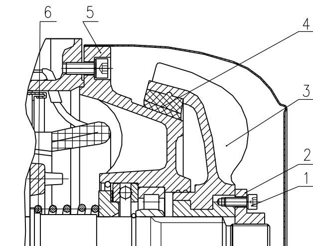
Схема регулировки тормозной системы
