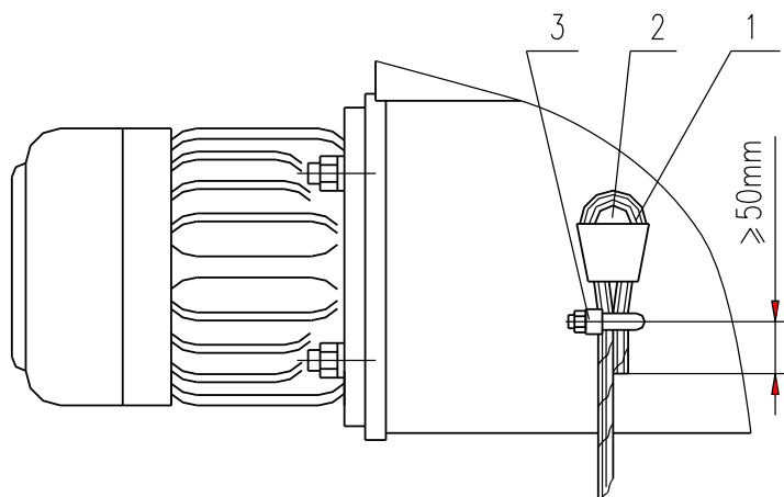
Проверка упругости каната
