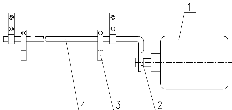
Схема концевого выключателя
